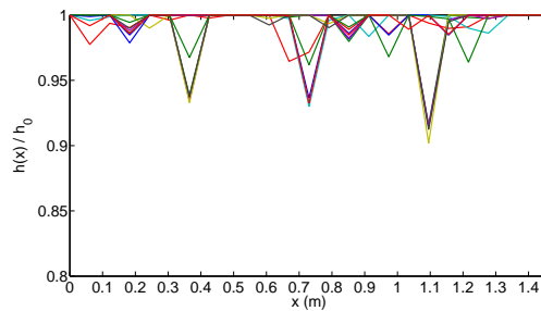
Figura 4: Identificação de danos das 10 simulações com o método ED para o Caso 2.
