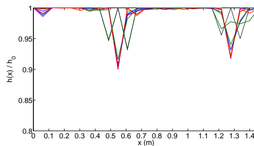
Figura 2: Identificação de danos das 10 simulações com o método ED para o Caso 1.
