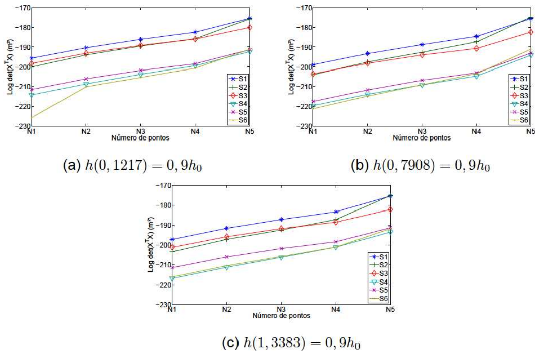
Figura 1: Determinante da matriz ( \mathbf{X}^T \mathbf{X} ) calculada para diferentes sensores e cenários de dano
