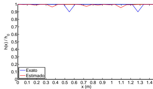
Figura 5: Identificação de danos obtida da média dos 10 resultados individuais do método ED para o Caso 2.
