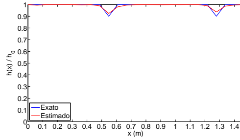
Figura 3: Identificação de danos obtida da média dos 10 resultados individuais do método ED para o Caso 1.
